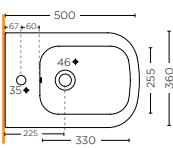
BIDET FILO MURO 50Q BACK TO WALL BIDET 50Q SMMX.30.F01Q
