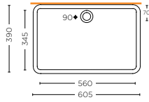
FORSAN LAVELLO 60 cm FORSAN SINK 60 cm
