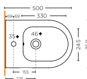
BIDET SOSPEO 50R WALL HUNG BIDET 50R SMMX.30.WO1R
