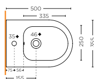
BIDET FILO MURO 50R BACK TO WALL BIDET 50R SMMX.30.FOIR
