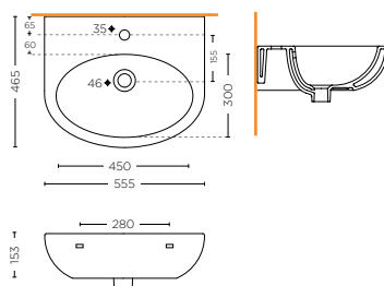
LAVABO 55 cm WASHBASIN 55 cm SDBD.10.04
