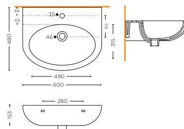
LAVABO 60 cm WASHBASIN 60 cm SDBD.10.03
