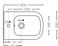
BIDET SOSPEO 50Q WALL HUNG BIDET 50Q SMMX.30.W01Q
