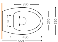
VASO SCARICO A PAVIMENTO WC S-TRAP SDBD.20.F10
