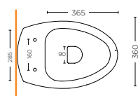
VASO NON FILO MURO NO BACK TO WALL WC SDBD.20.F02
