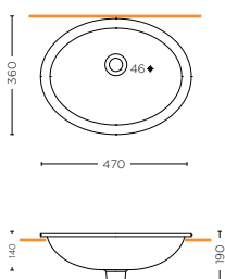
LAVABO SOTTOPIANO OVALE DA INCASSO 47 cm OVAL UNDER COUNTER WASHBASIN 47 cm
