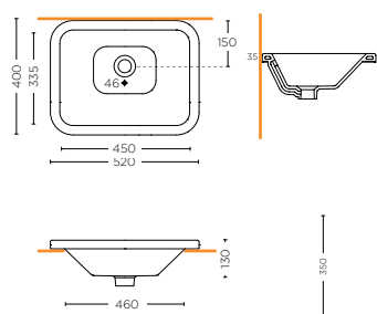
LAVABO DA INCASSO 52 cm * COUNTERTOP WASHBASIN 52 cm SMMX.10.21
