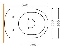
VASO SCARICO A PAVIMENTO WC S-TRAP SECO.20.F10
