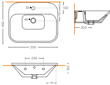
LAVABO 55 cm WASHBASIN 55 cm SMMX.10.19
