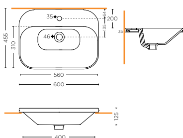
LAVABO DA INCASSO 60 cm * COUNTERTOP WASHBASIN 60 cm SMMX.10.20
