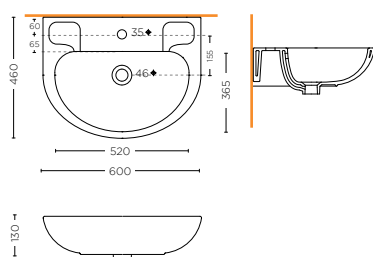
LAVABO 60 cm WASHBASIN 60 cm SECO.10.03
