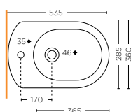
BIDET BIDET SECO.30.F10
