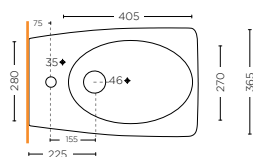
BIDET BIDET SMAJ.30.F01
