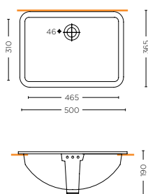
LAVABO SOTTOPIANO RETTANGOLARE DA INCASSO 50 cm RECTANGULAR UNDER COUNTER WASHBASIN 50 cm
