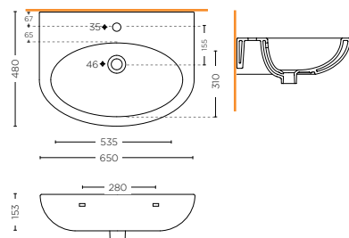
LAVABO 65 cm WASHBASIN 65 cm SDBD.10.01
