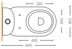
VASO MONOBLOCCO CON CASSETTA SCARICO A PAVIMENTO CLOSE COUPLED WC WITH CISTERN S-TRAP SECO.20.C10 / SECO.28.10
