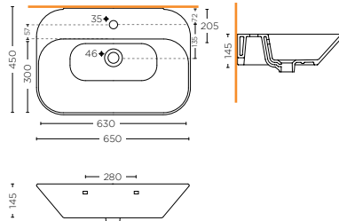
LAVABO 65 cm WASHBASIN 65 cm SMMX.10.01
