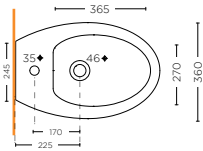
BIDET SOSPESO WALL HUNG BIDET SDBD.30.W01
