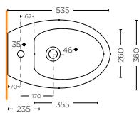
BIDET FILO MURO BACK TO WALL BIDET SDBD.30.F01
