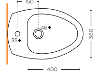
BIDET NON FILO MURO NO BACK TO WALL BIDET SDBD.30.F02
